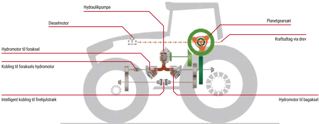
Diagram, der viser designet af Fendt VarioDrive.
