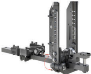
Barra de tiro extensible con orificio 30 mm (A192)
