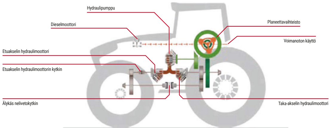
Kuvassa on esitetty Fendt VarioDrive -voimansiirron osat.
