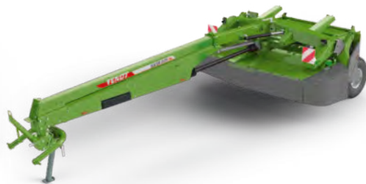
Getrokken maaiers met transportonderstel Grote flexibiliteit met tanden- of rollenkneuzer Werkbreedte 3,00 m
