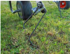
Graset plukkes opp med den 7,5 cm lange kroken på Fendt Performance-tindene.
