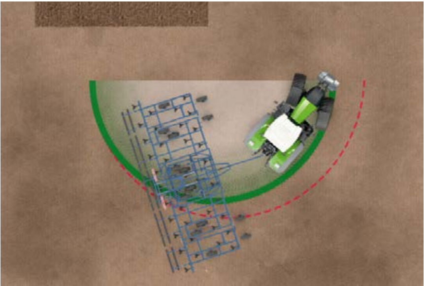
Liten svingradius takket være "pull-in turn"-effekten, f.eks. 6,1 m for Fendt 930 Vario med standard dekk.
