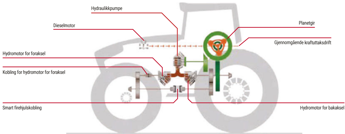
Diagram som viser designet til Fendt VarioDrive.
