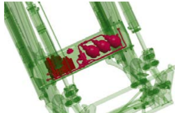
Alla hydraulkomponenter är monterade i tvärbalken och är därför helt skyddade mot smuts och mekaniska skador.
